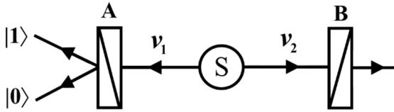
Рис.7. Схема экспериментальной установки
